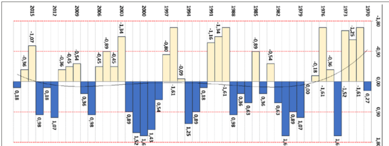
FIGURE 6 : Indice régional calculé à partir des écarts centrés réduits des cumuls annuels de pluviométrie pour dix stations de l'ex région Haute-Normandie
